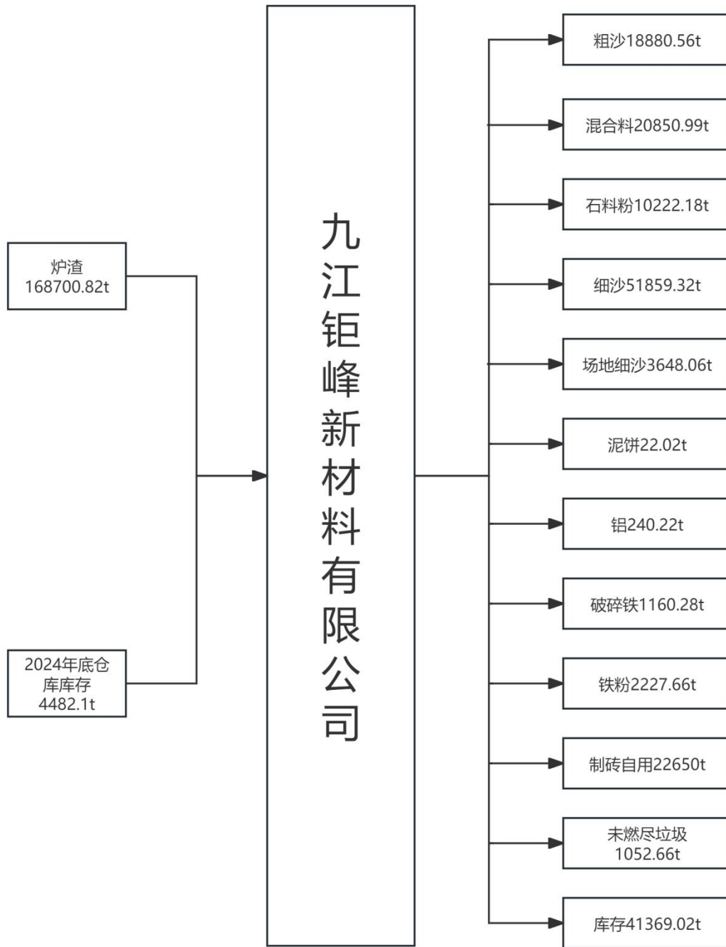
图 7.4-1 炉渣物料平衡图
