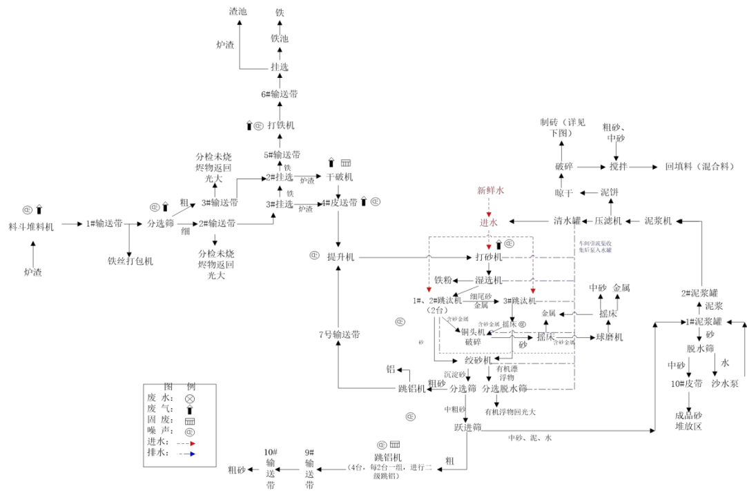
图 4.1-1 项目砂、道路垫层及回填料（混合料）工艺流程图
